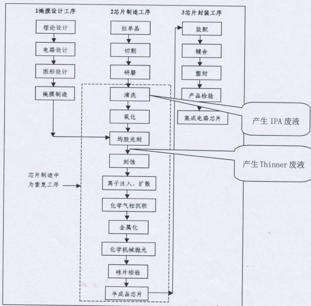
完整的集成电路生产简化工艺流程
